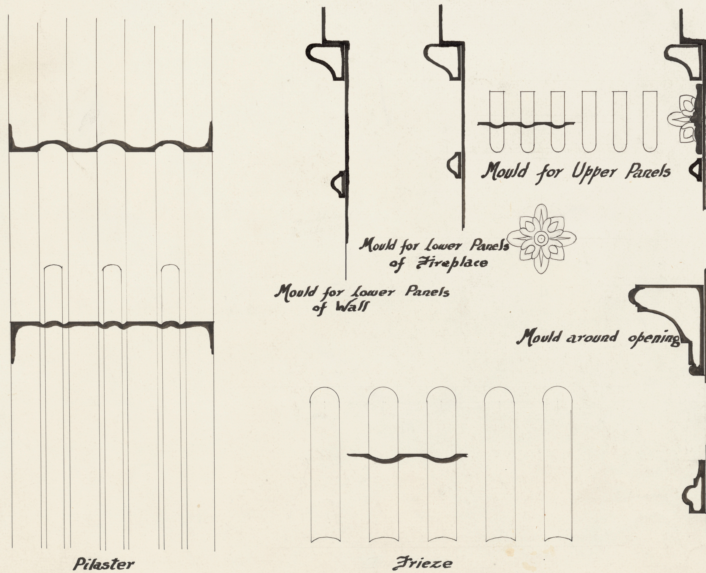
ELEVATION
