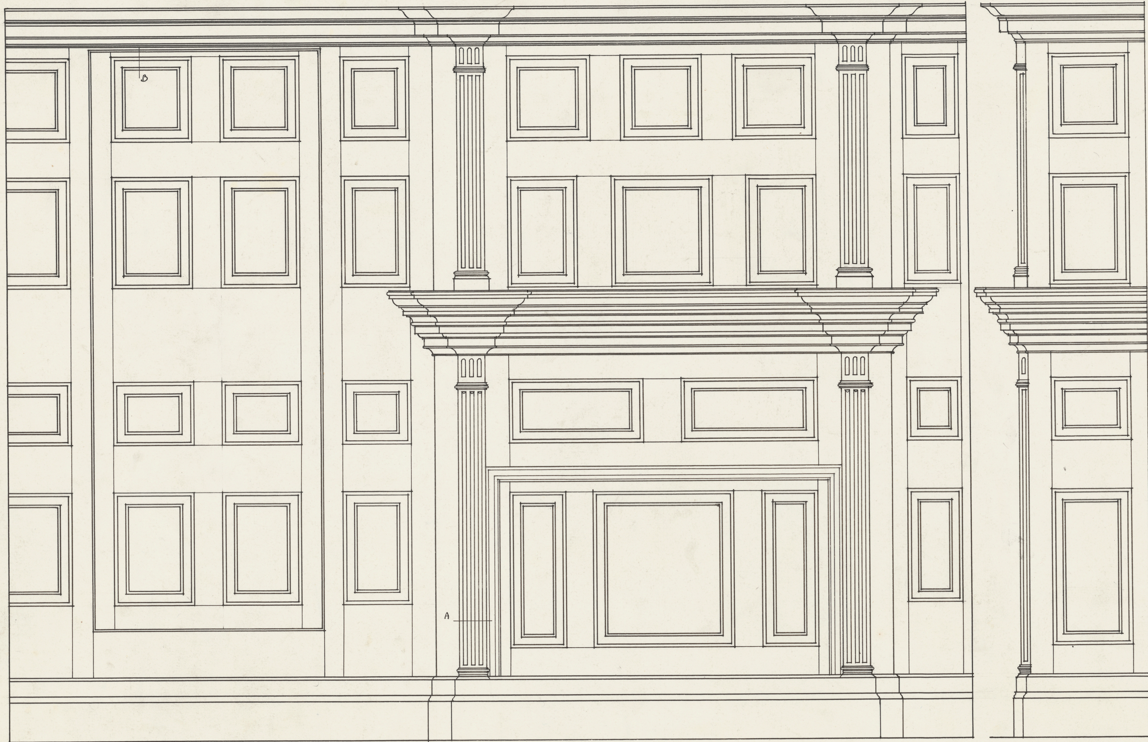
Elevation
